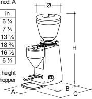
ELECTRONIC GRINDER-DOSER MINI mod. A
